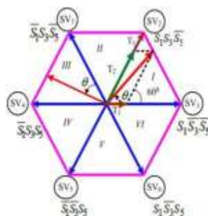
Fig. 3. SVPWAM for VSI.
